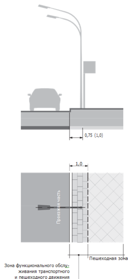
Вариант2 Шириназоны —1,0м
