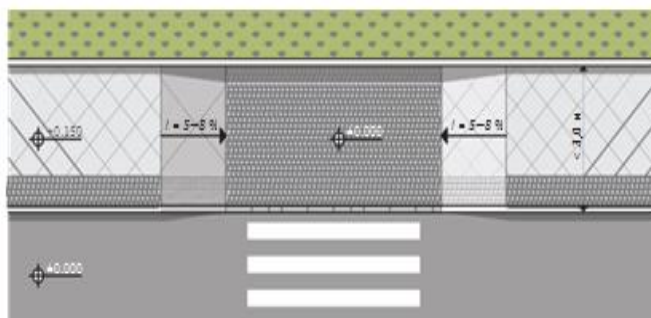
Схема 4–2. Пример организации предупреждающих покрытий при помощи изменения цвета, фактуры и типа укладки
