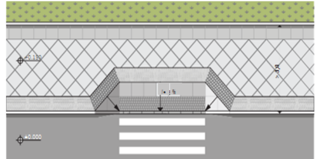
Схема 3–2. Пример организации предупреждающих покрытий при помощи изменения цвета, фактуры и типа укладки
