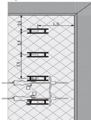
Велопарковка, перпендикулярная фасаду
