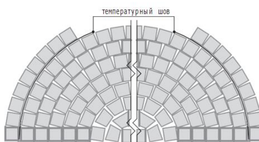
Тип 8. Радиальная кладка Используемая плитка – брусчатка
