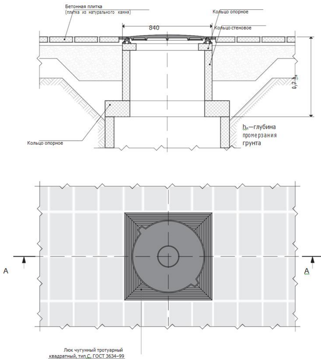
Сечение А-А
