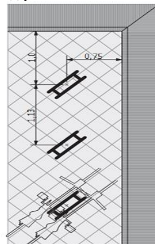
Велопарковка, расположенная под углом 45°
