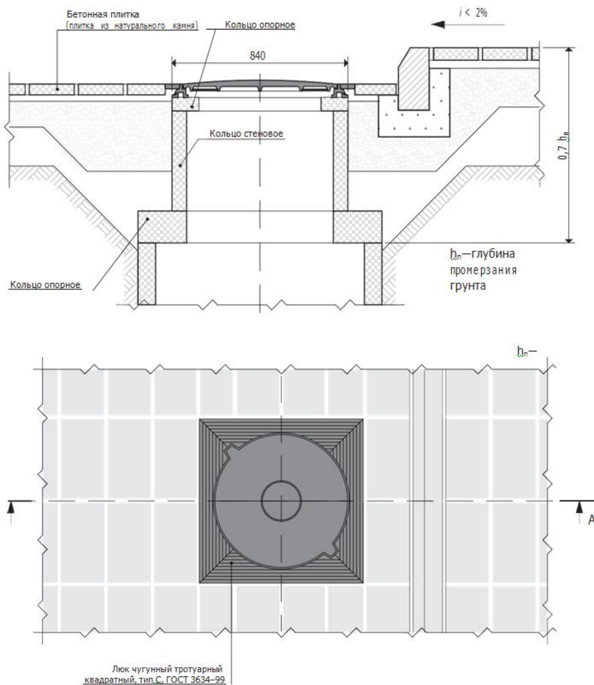
Сечение А-А
